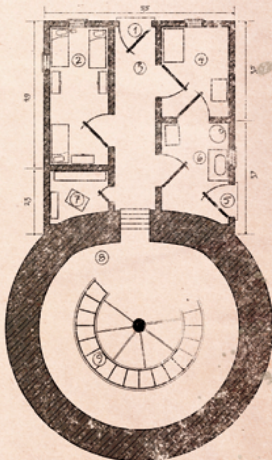
PLANTA BAIXA
